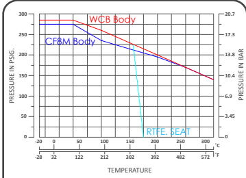
1/2" ~ 2" ( DN15 ~ DN50 )
